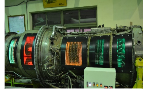
PW J-57 發動機
